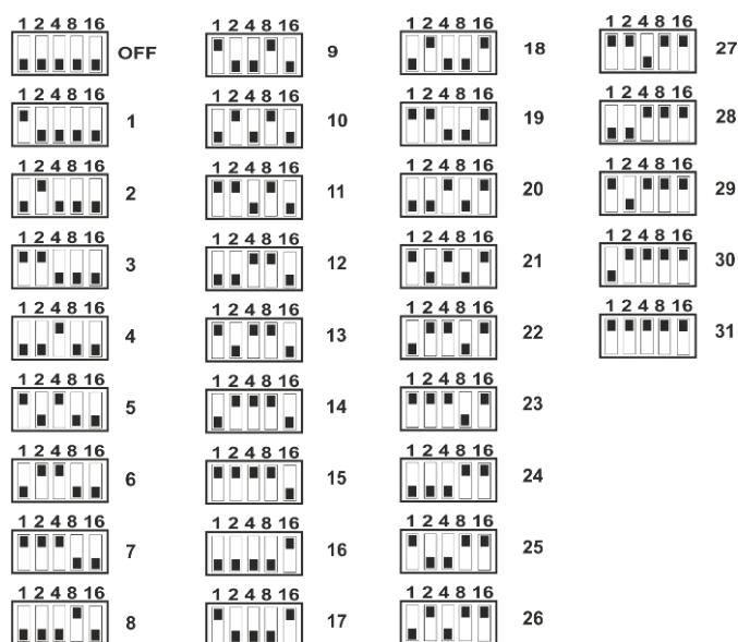
Рис. 2. Назначение адреса адаптера зоны СДК-037
