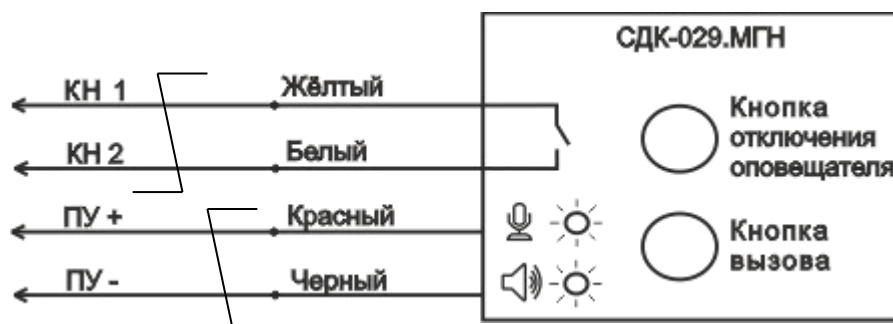
Рис. 3. Подключение СДК-029.МГН
