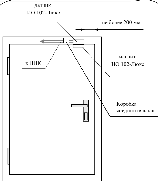
Рисунок 2. Пример установки извещателя для охраны дверного проема
